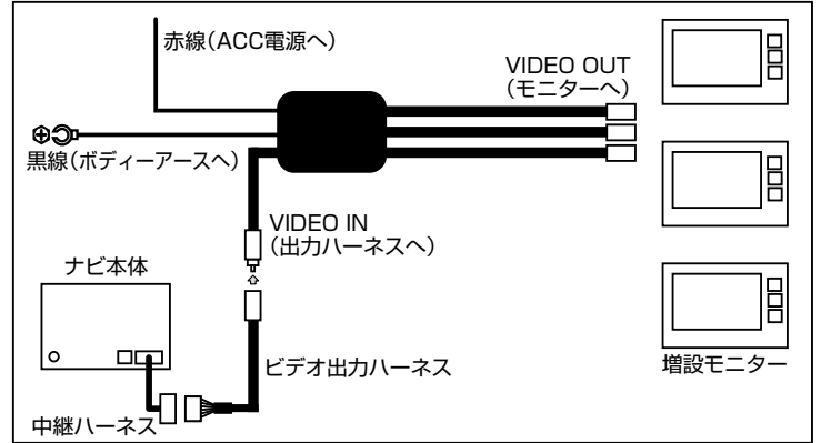
接続概要図
