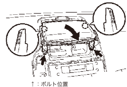
↑: ボルト位置
