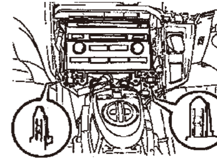
図8 オーディオユニット取り外し (分配器の電源取得のために外します)
