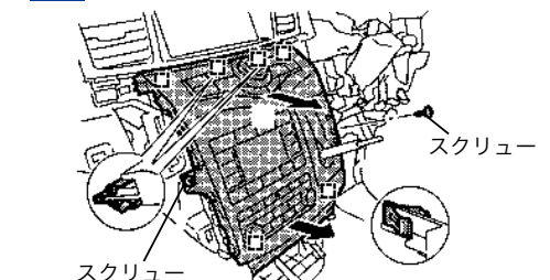
図12 オーディオパネル取り外し
