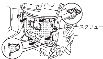
図7 インパネクラスター取り外し
