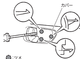
●:ツメ
