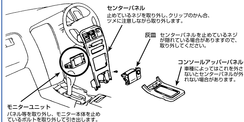
図1 パネル類取り外し、モニター取り外し
