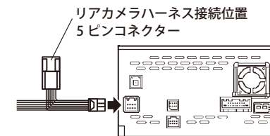
リアカメラハーネス接続位置 5ピンコネクター モニター裏の形状は図と異なる場合があります。
