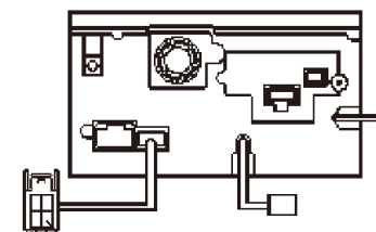
リアカメラハーネス接続位置 4ピンコネクター （ナビ付属中継ハーネス）
