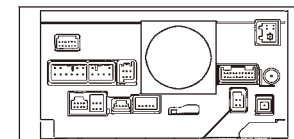
リアカメラハーネス接続位置 4ピンコネクター
